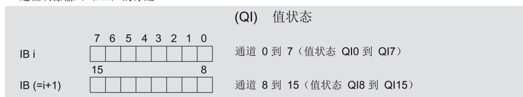
图 4-1 组态为带值状态的 16 通道 DQ 16x24VDC/0.5A ST 的地址空间
