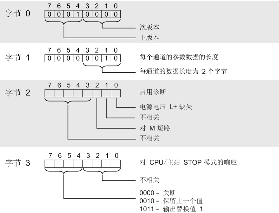
图 B-1 数据记录 64 的结构： 字节 0 到 3
