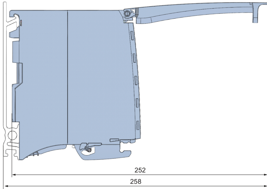
图 A-2 DQ 16x24VDC/0.5A ST 模块的尺寸图，带开放式前盖的侧视图
