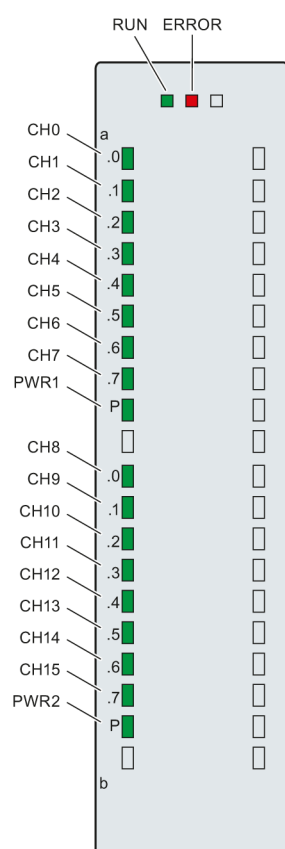
图 5-1 LED 模块的指示灯 DQ 16x24VDC/0.5A ST
