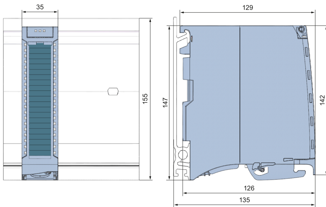
图 A-1 DQ 16x24VDC/0.5A ST 模块的尺寸图
