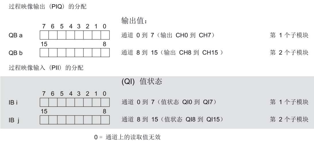
图 4-2 组态为带值状态的 2 x 8 通道 DQ 32x24VDC/0.5A ST S QI 的地址空间
