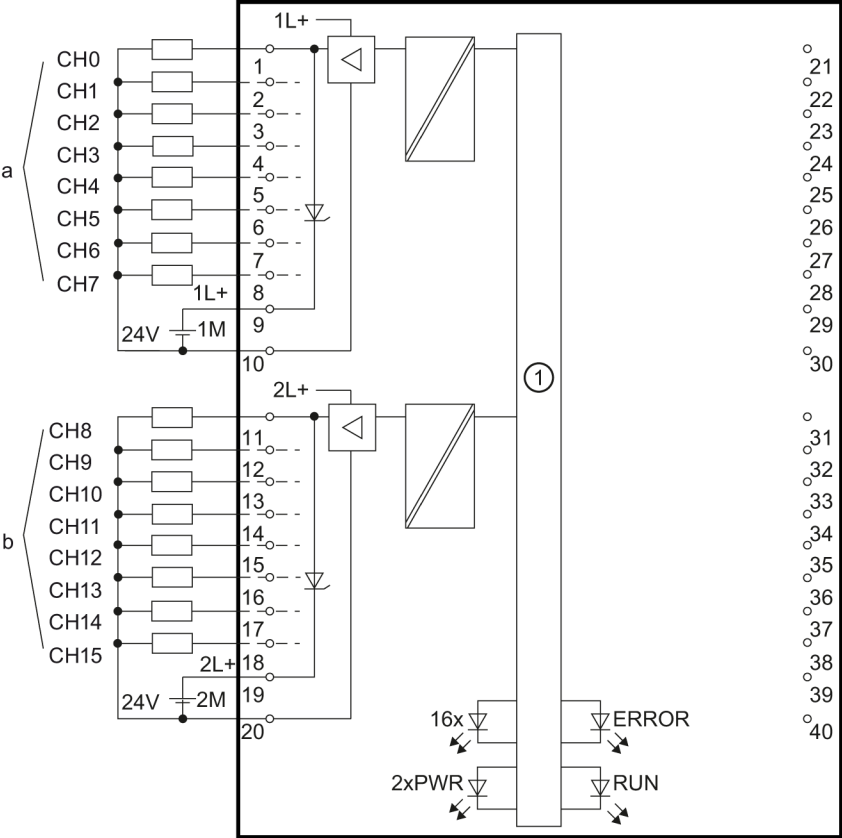
图 3-1 方框图和端子分配
