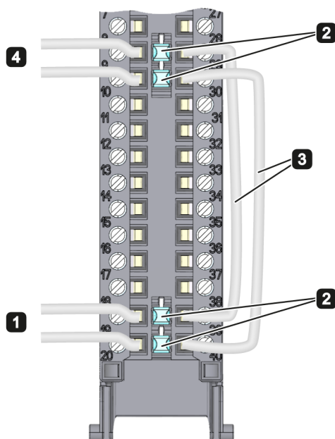
图 3-2 使用电位跳线
