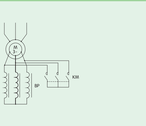
图2 单组接法
