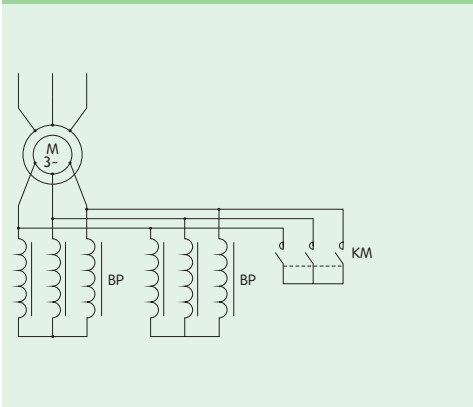
图3 二组并联(2并)接法
