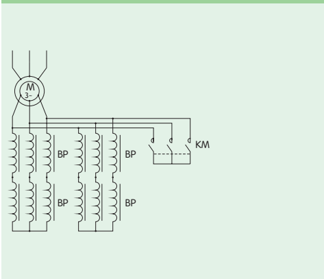
图5 二串二并接法
