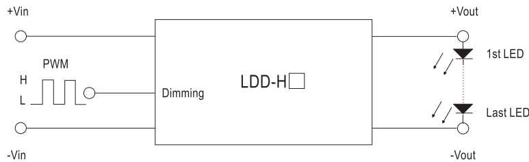
图-1 12VDC输入, 1~3 LEDs(Vf=3V)
