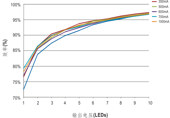
图-3 36VDC输入, 1~10 LEDs(Vf=3V)
